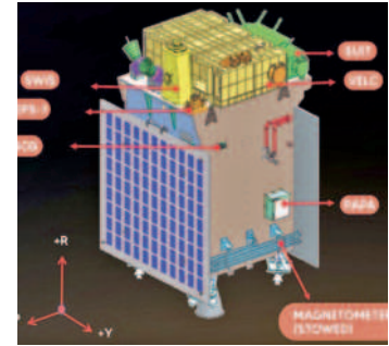
శ్రీహరికోట (తద), జనవరి 25 ప్రభాతవార్త భారత అంతరిక్ష పరిశోధన సంస్థ సూర్య పరిశోధనల కోసం ప్రయోగించిన ఆదిత్య ఎల్1 ఉపగ్రహంలో మాగ్నెటిక్ మీటర్ బూమ్ విజయవంతంగా పనిచేస్తోంది. ఇలా గరువారం ఎల్1లో ఈ మేరకు ప్రకటించింది. శ్రీహరికోట నుంచి ఆదిత్య ఎల్1 ప్రయోగించినప్పటి
